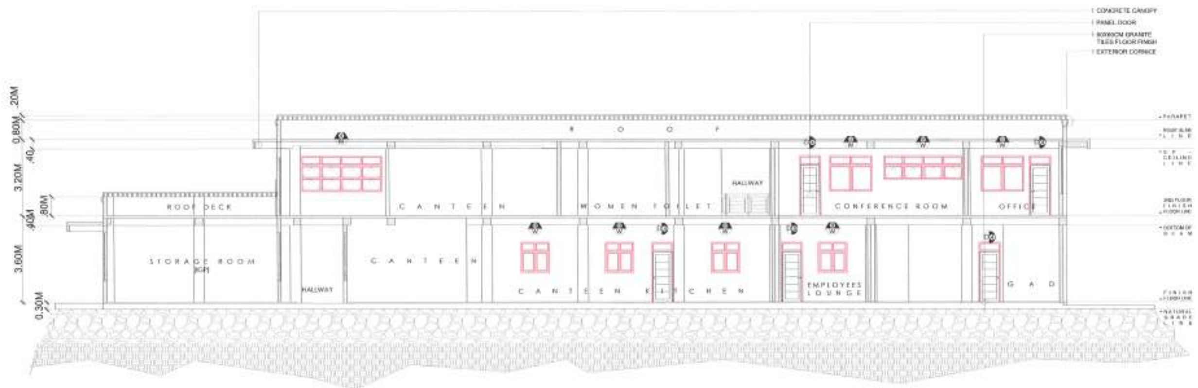
1 LONGITUDINAL SECTION A - 9 SCALE: 1:200 MTS.
