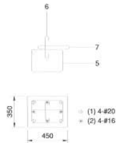
SECTION 1-1 (C25) (SCALE 1:25)
